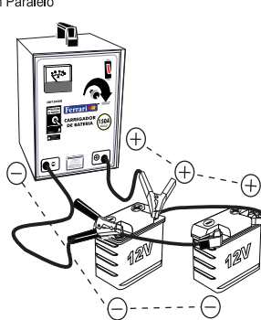
Recarregando 2 Baterias em Paralelo
